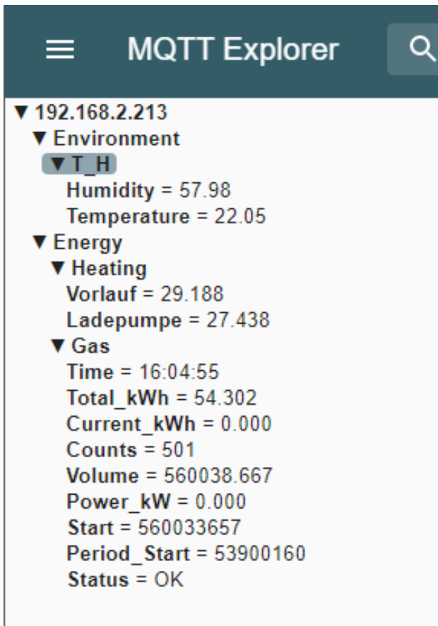
Abbildung 2: MQTT Topics
